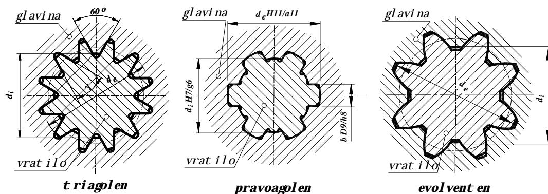
Sl.6.14 Popre~en presek na `leben spoj
